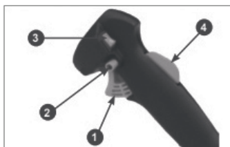
Рис. 8 1 - Рычаг газа, 2 - Фиксатор рычага газа, 3 - Выключатель зажигания, 4 - Рычаг предохранительный
