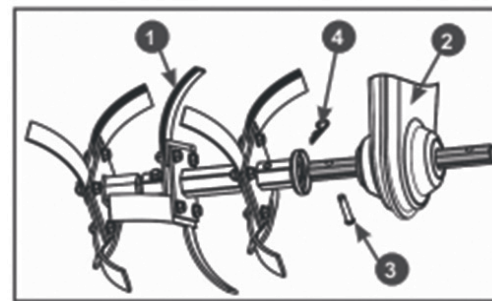
Рис. 10 Установка собранной фрезы на вал редуктора
