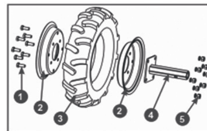
Рис. 15 Сборка колеса
