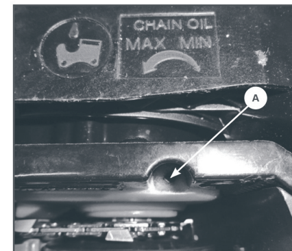
Рис. 12 Положение регулировочного винта подачи масла
