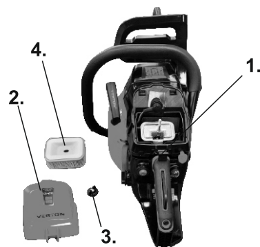
Рис. 20 Обслуживание воздушного фильтра
