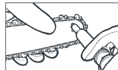
Рис. 30 Смазывание подшипника ведомой звездочки шины
