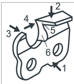
Рис. 29 Части режущего звена цепи
