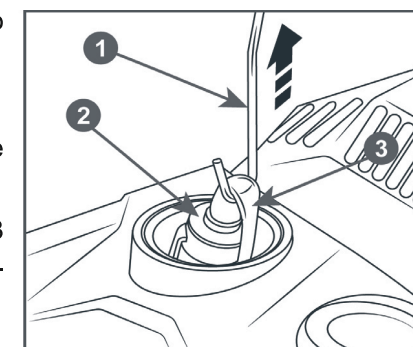
Рис. 21 Обслуживание топливного фильтра 1 - Фильтр топливный; 2 - Крючок; 3 - Шланг
