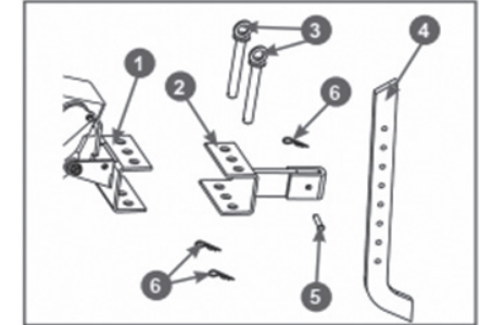
Рис. 11 Установка сошника
