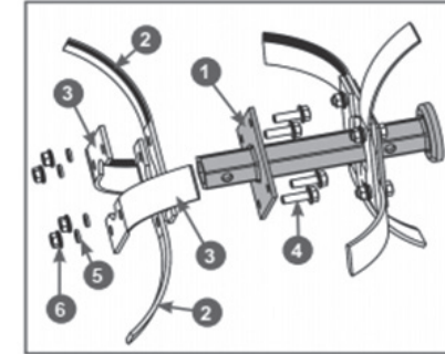
Рис. 7 Установка ножей на внешний фланец основной секции оси фрезы
