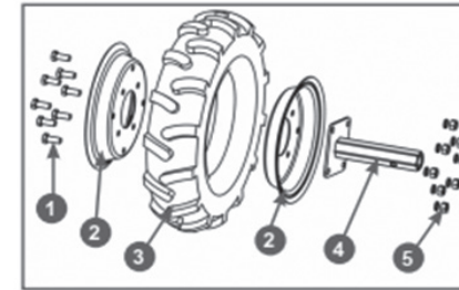
Рис. 15 Сборка колеса
